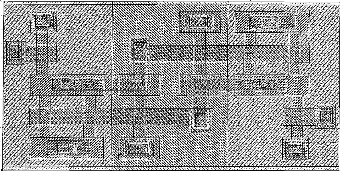
Fig 3.5: FinFET SRAM layout.
